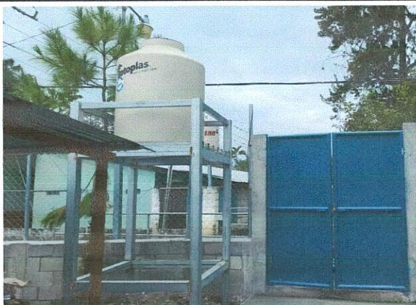
Foto 3: Área finalizada en la que se realizó el mejoramiento e instalación de un tanque elevado destinado al almacenamiento de agua.
