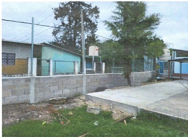
Foto1: Área finalizada en la que se realizó el mejoramiento de los 80 metros cuadrados de la losa de patio del lado Sur.
